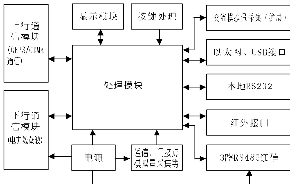
图 1 原理框图
