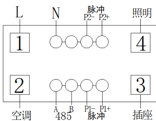
一进三出接线图
