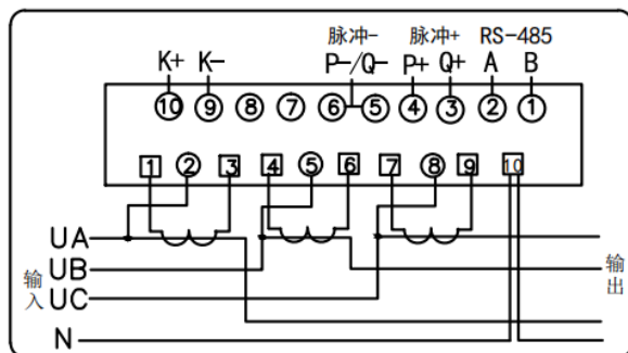
(a) 小电流互感式接线图
