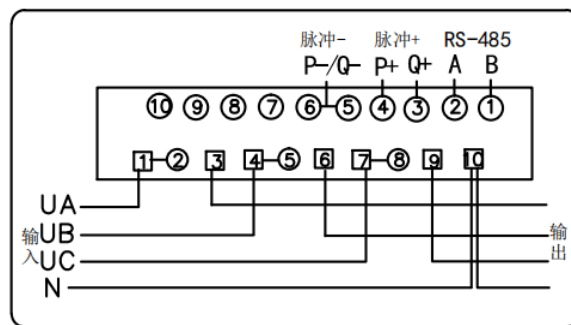
(b) 大电流直通式接线图
